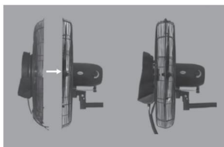
Συναρμολόγηση της λεπίδας, της πίσω σκάρας, του μοτέρ του ανεμιστήρα και του σωλήνα.
