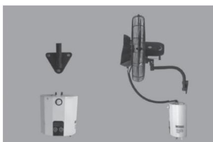
Συναρμολόγηση της πρόσοψης. Σύνδεση του καλωδίου και του σωλήνα του δίσκου υδρονέφωσης.
